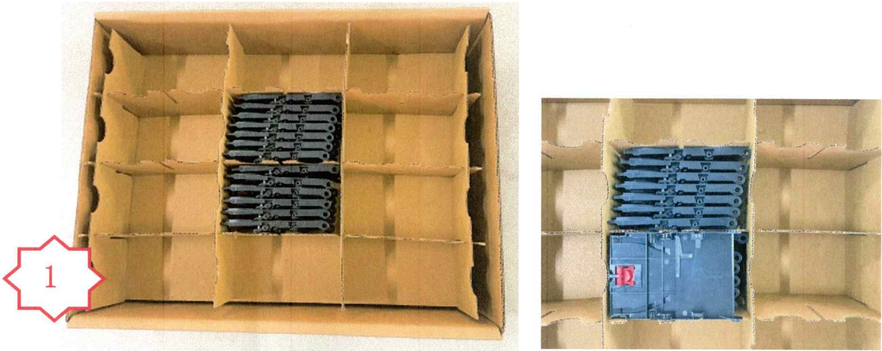
图一，每格 7pcs，每层 12 格，每层 84pcs，共 2 层，满箱 168pcs
