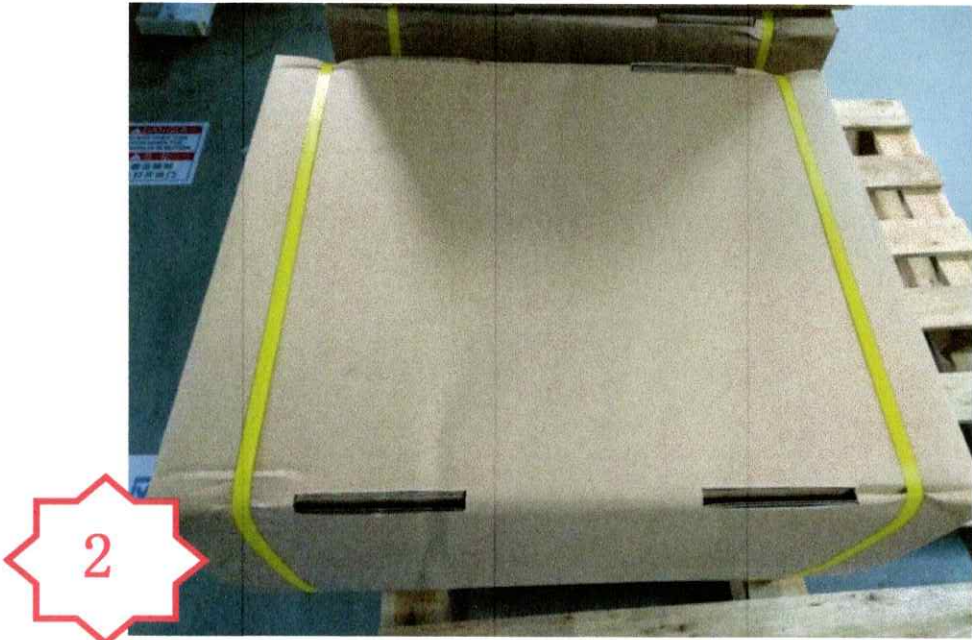
图二，确认 PA2725 无漏装后，将 26 的内箱与外箱配合并打包装带待出货
